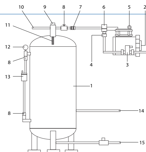
Inkopplingschema för kompressor-anläggning inklusive luftningsanordning
